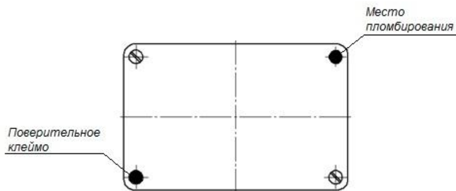
Рисунок Ж.1 – Пломбирование крышки ПР (исполнение без индикации)
