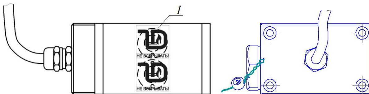
Продолжение рисунка Ж.3 – Схема пломбирования расходомера
