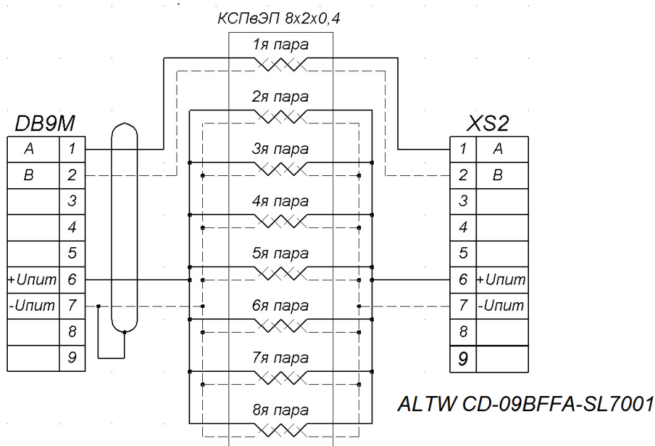
Рисунок Л.2 – Схема распайки кабеля КСПвЭП 8×2×0,4 для подключения ВТ и ПР
