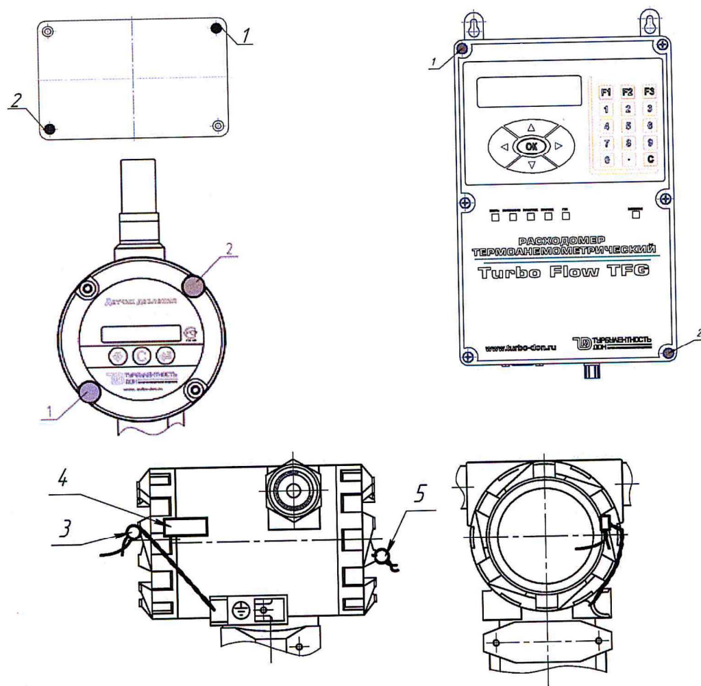
Рисунок 2 - Схема пломбирования ПП и РП расходомера
